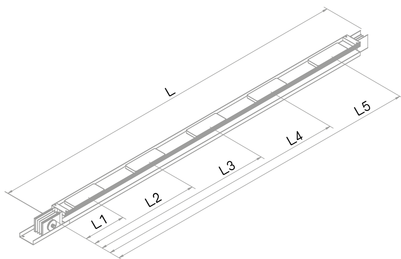
Рис. 2 Прямая секция
