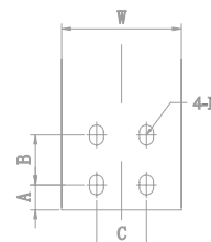
Рис. 10 Присоединительные размеры контактных площадок присоединительных секций
