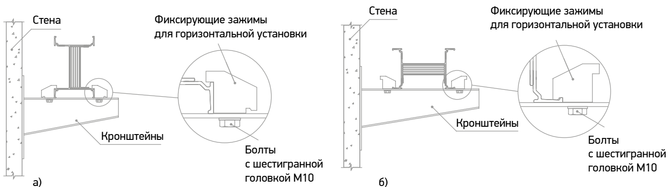
Рис. 18 Горизонтальная установка шинопроводов (опорная стена): а) установка «на ребро» б) установка «плашмя»
