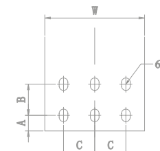
Рис. 10 Присоединительные размеры контактных площадок присоединительных секций
